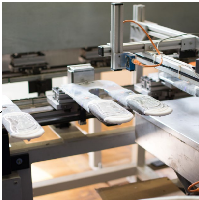
Beschichtung VABS-Sohle
